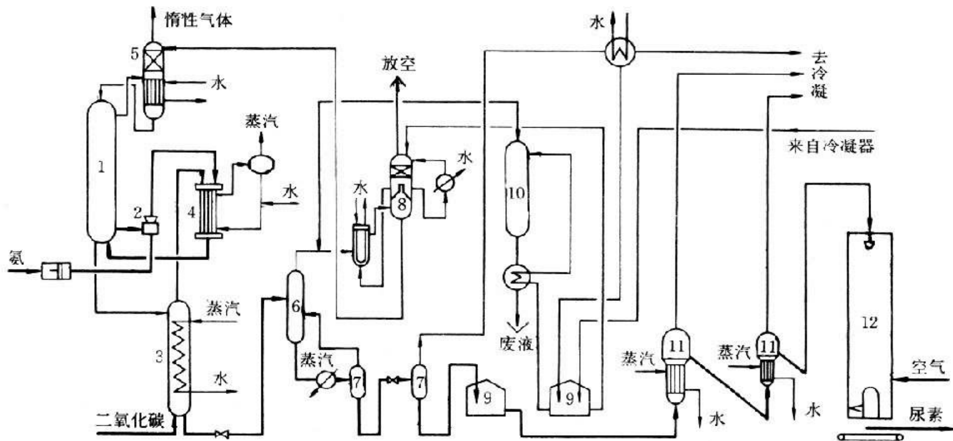
图2 二氧化碳气提法尿素生产流程
